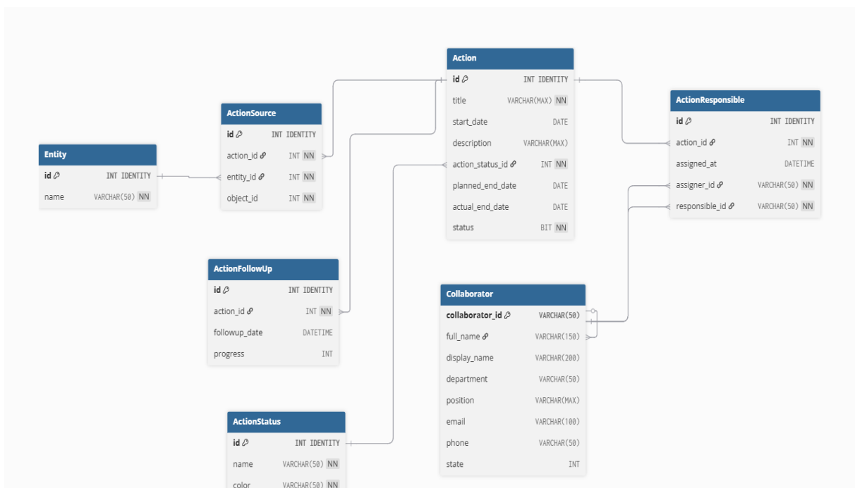
Figure 13 : Conception de la base de données pour le module gestion des actions
