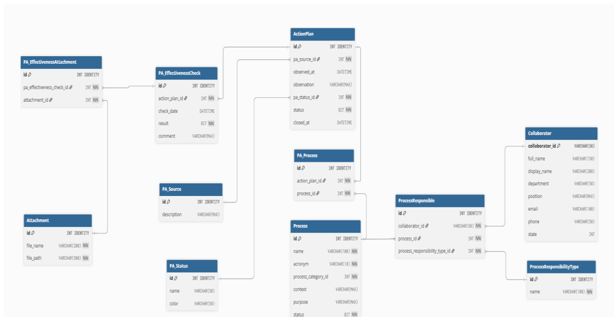
Figure 12 : Conception de la base de données pour le module plan d'action
