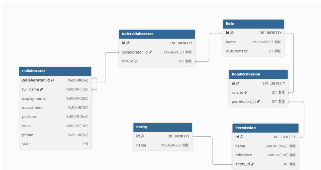
Figure 10 : Conception de la base de données pour le module de gestion des autorisations
